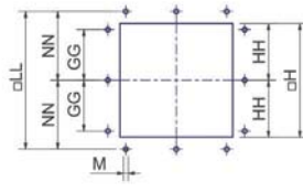
Фланец горелки
